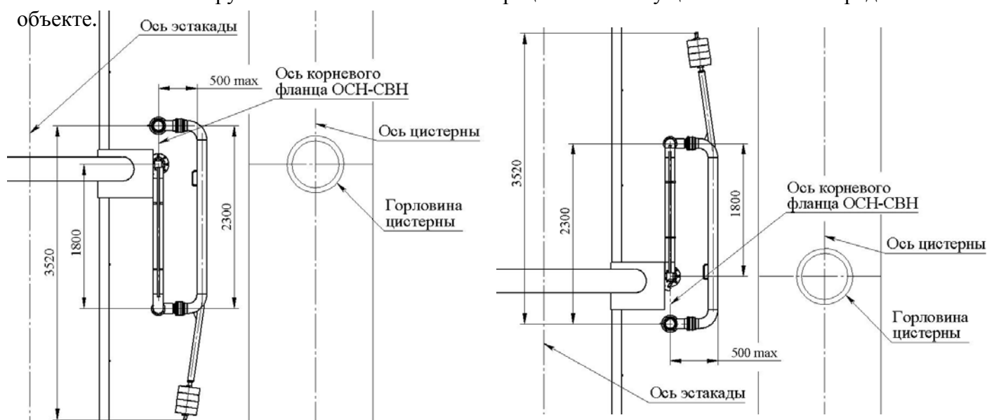
Рис. 4. Правое и левое парковочные положения ОСН-СВН-100-У-6-НН на ж/д эстакаде.
