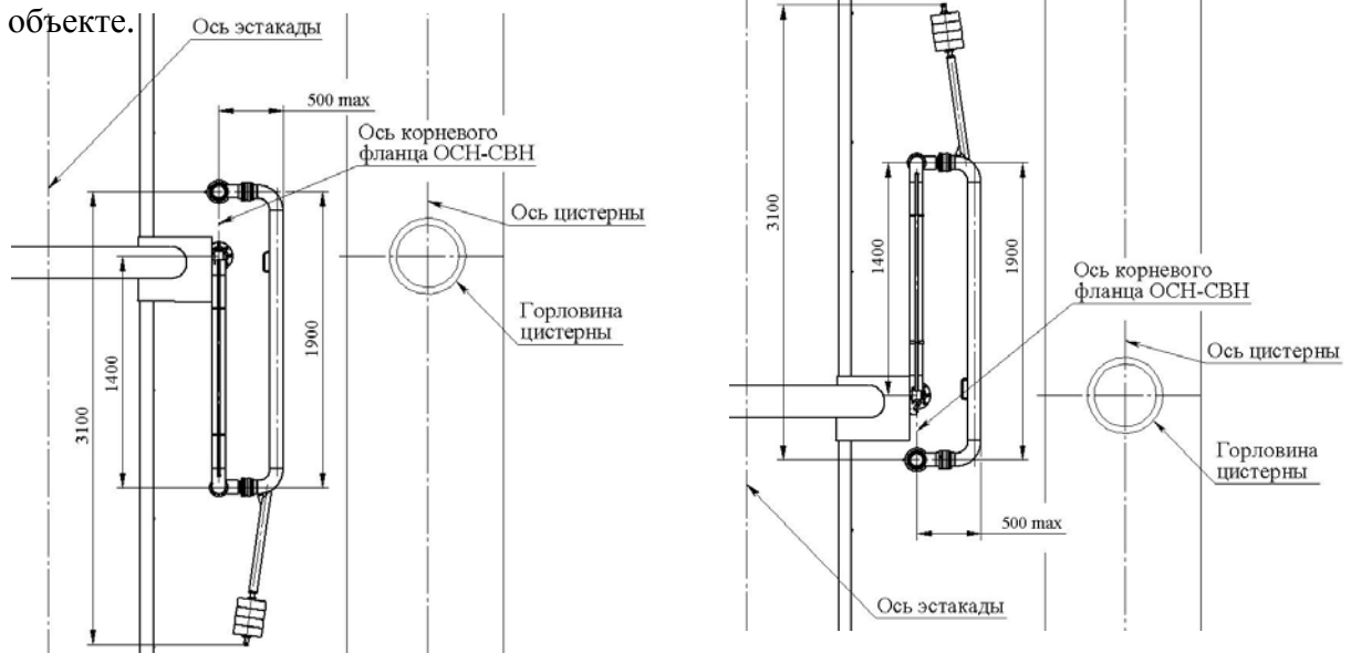
Рис. 4. Правое и левое парковочные положения ОСН-СВН-100-К-З-4-НН на ж/д эстакаде.
