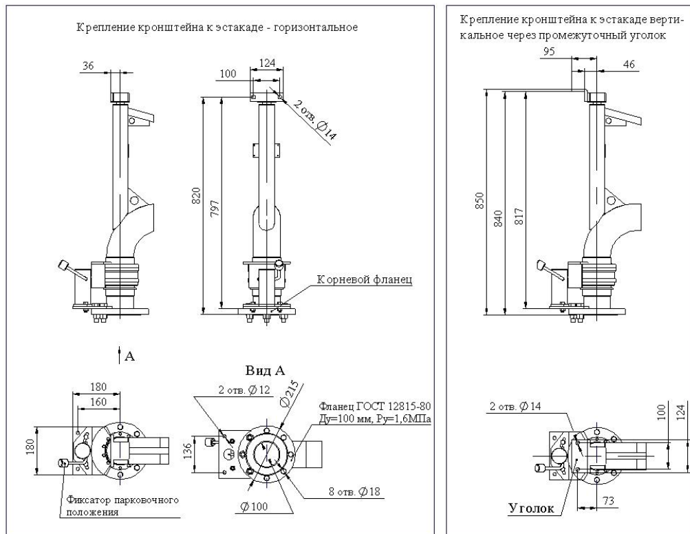
Рис. 3. Установочные размеры ОСН-СВН-100-К-З-4-НН.
