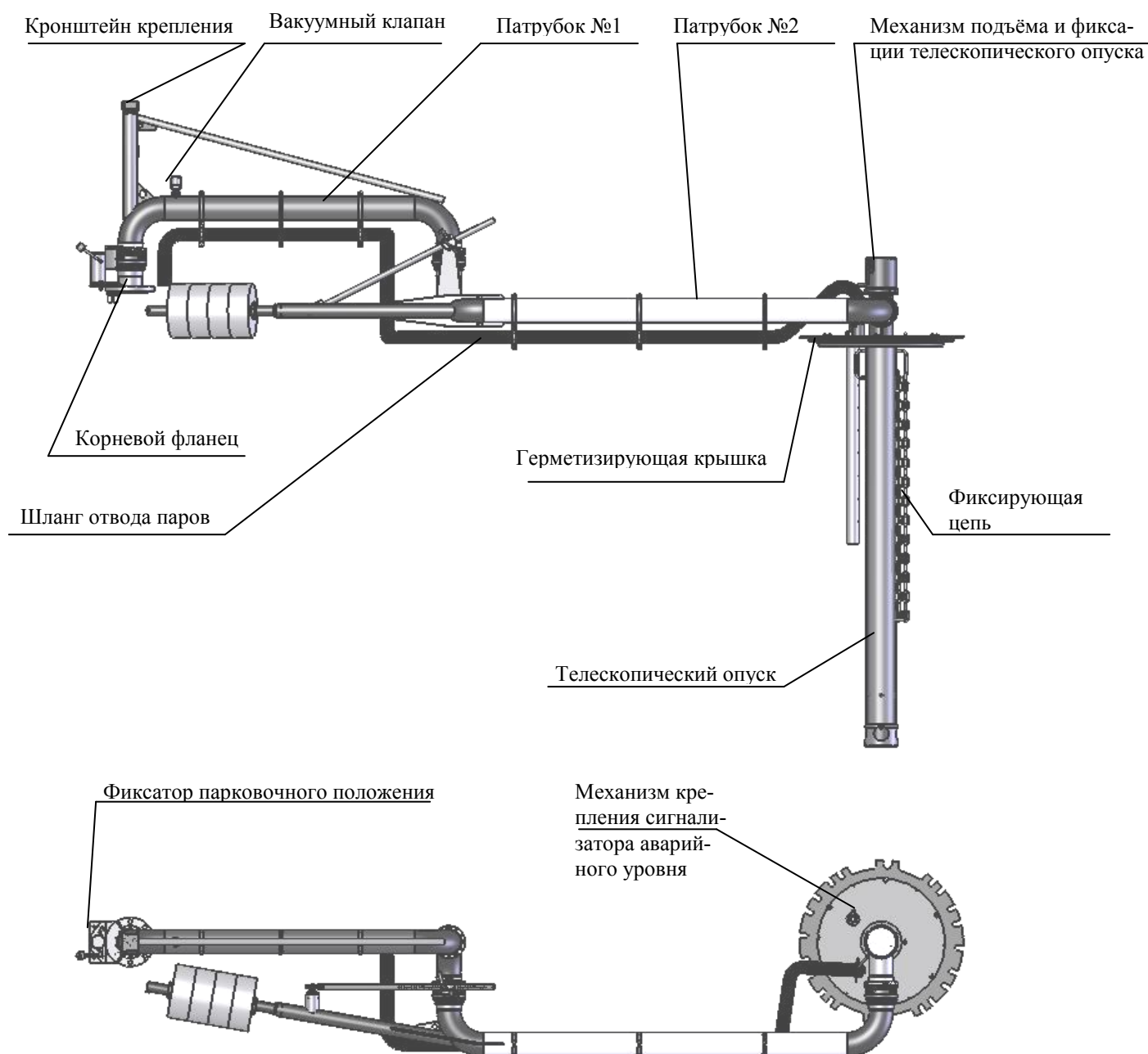
Рис. 1. Конструкция стойка верхнего налива ОСН-СВН-100-К-3-4-НН.
